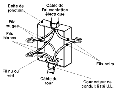
Figure A Neutre mis à la terre
