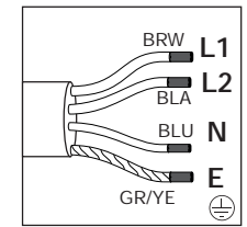
2 N AC 220-240 V / 380-415 V
