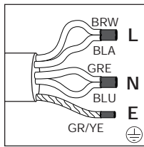
1 N AC 220-240 V
