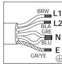
2 N AC 220-240 V / 380-415 V
