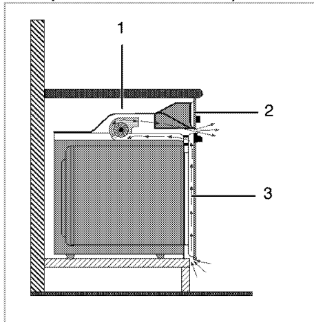
1 Chladiaci ventilátor
