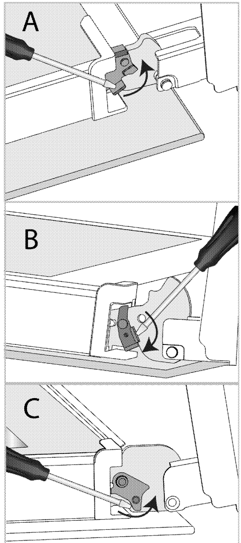
Scharniergegrendeling - gesloten positie
